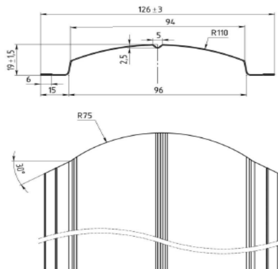
Профиль «Штакетник «Европланка»
